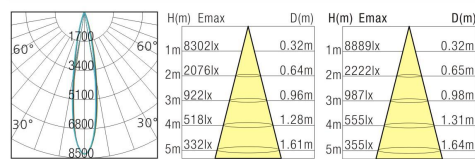
24° 3000K 4000K
