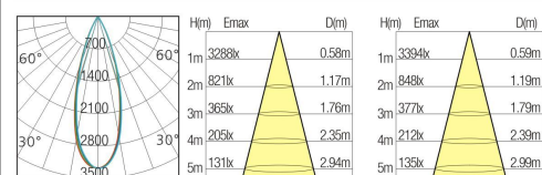
36° 2700K 3000K
