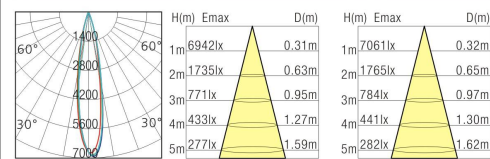
24° 2700K 3000K
