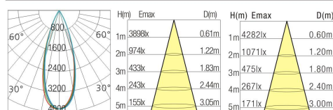
36° 3000K 4000K
