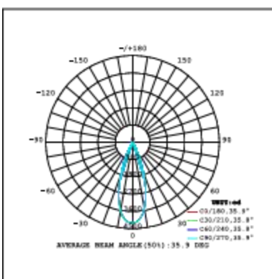
20W CRI90 36°
